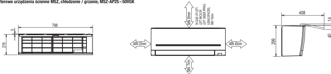
Inwerterowe urządzenia ściennie MSZ, chłodzenie / grzanie, MSZ-AP25-50VGK
