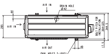
Inwerterowe urządzenia zewnętrzne SUZ, chłodzenie / grzanie, SUZ-M25/35VA
