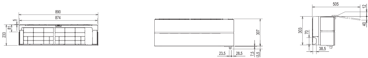
Urządzenia ściennie MSZ Diamond, chłodzenie / grzanie, MSZ-LN18-60VG2 R/W/B
